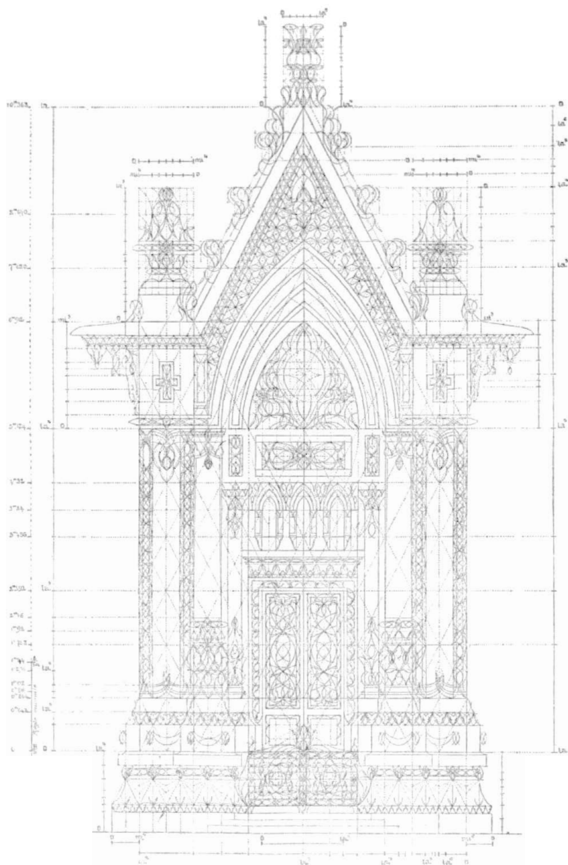
GRANDE CHAPELLE. — Détail du Porche et Porte d'entrée (Style ogival). — Accord La, Cl, Mi.
