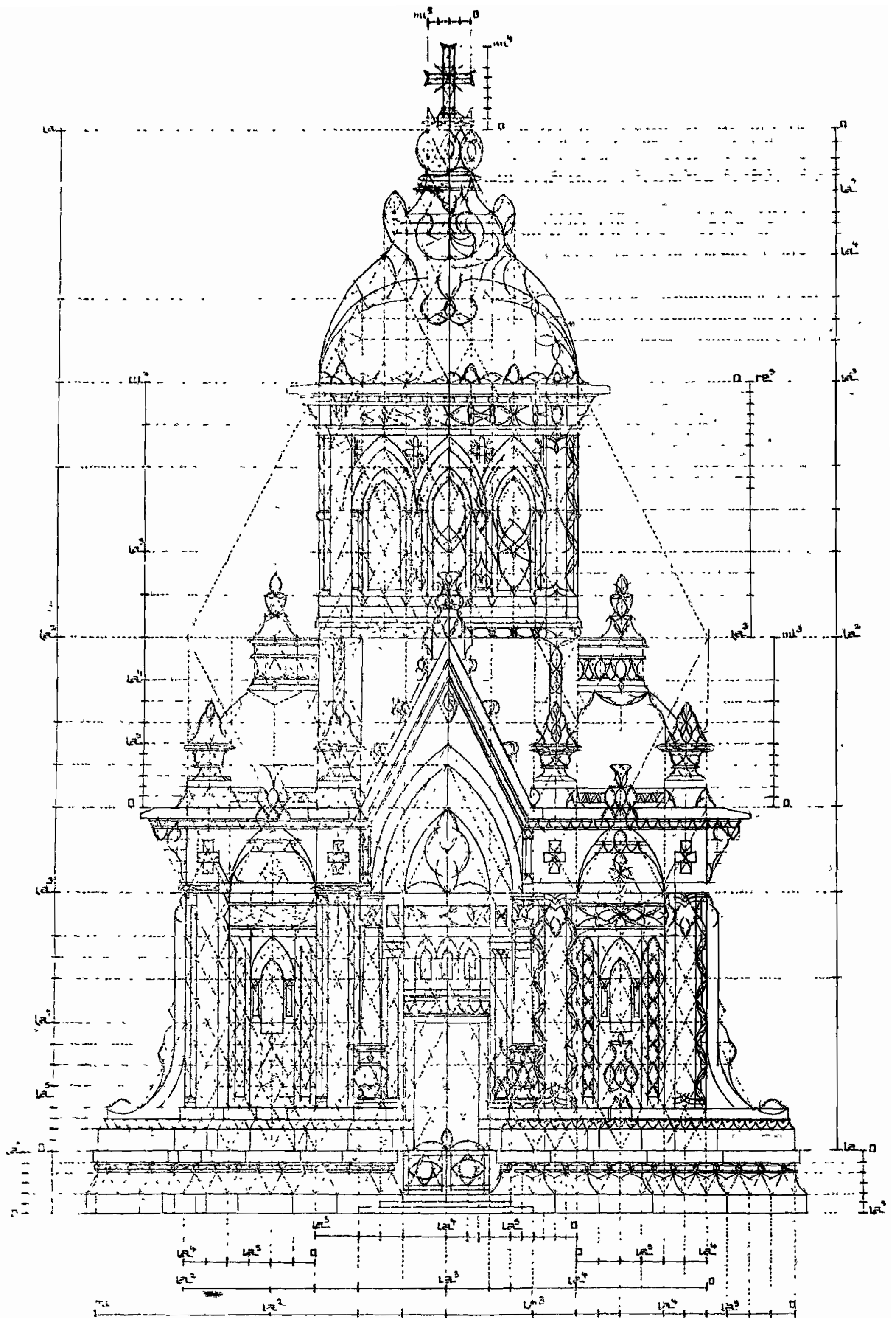
GRANDE CHAPELLE. — Façade (Style ogival). — Accord La, U, Mi.
