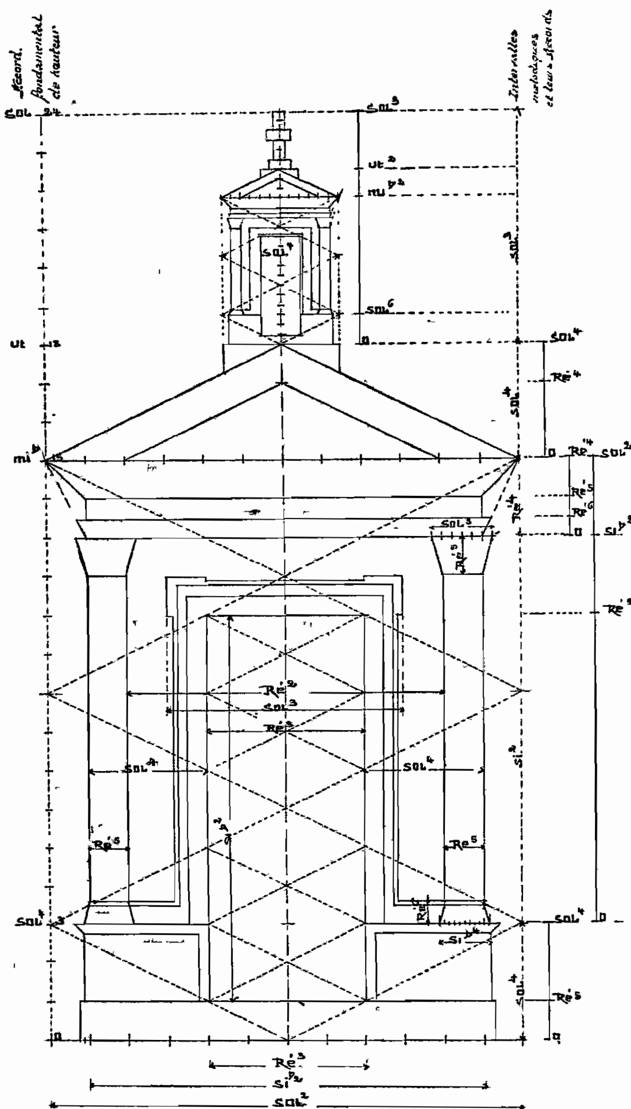
Type de Charpente musicale
