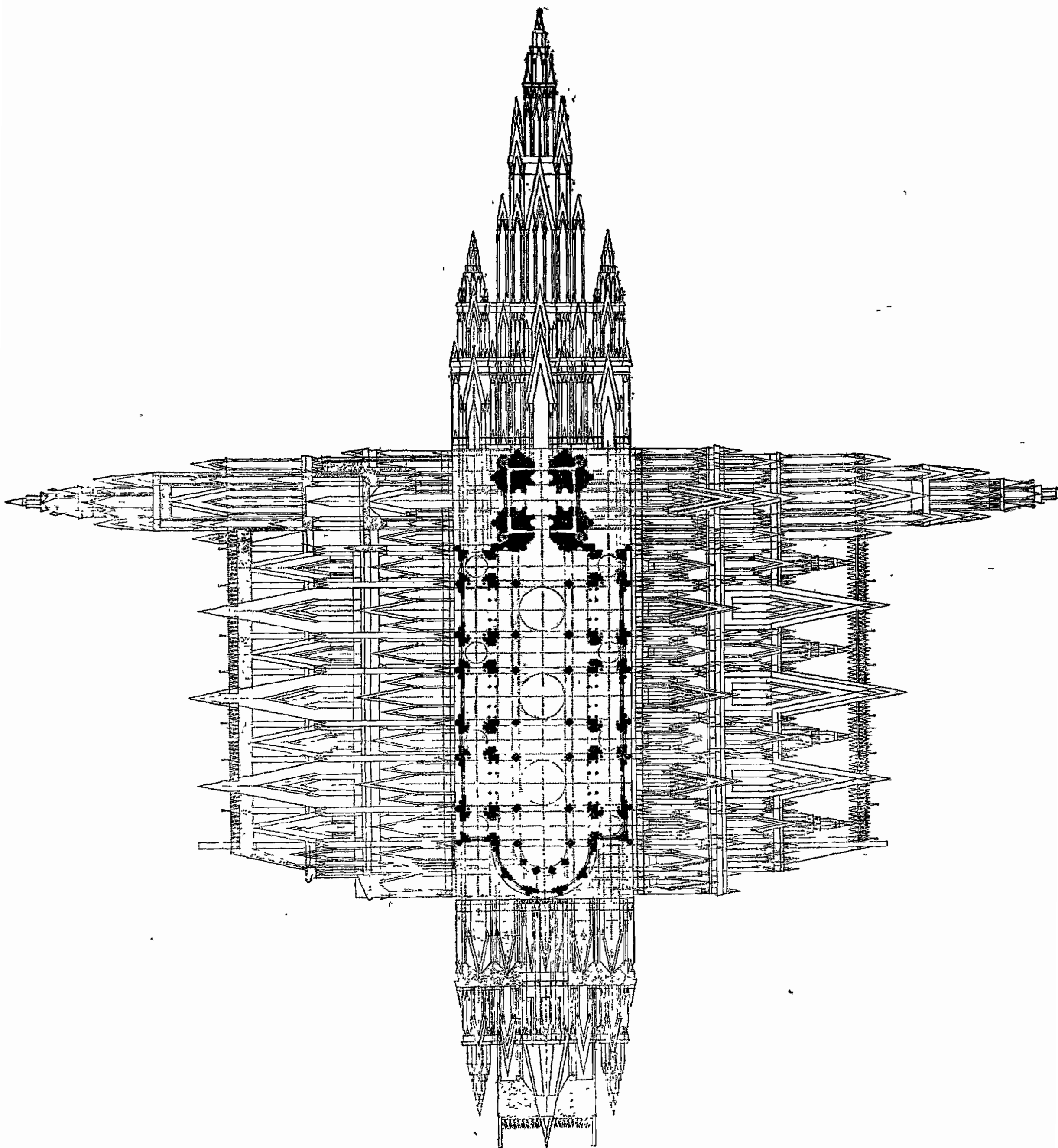
ÉGLISE. — Charpente musicale des plan coupes et élévations.
