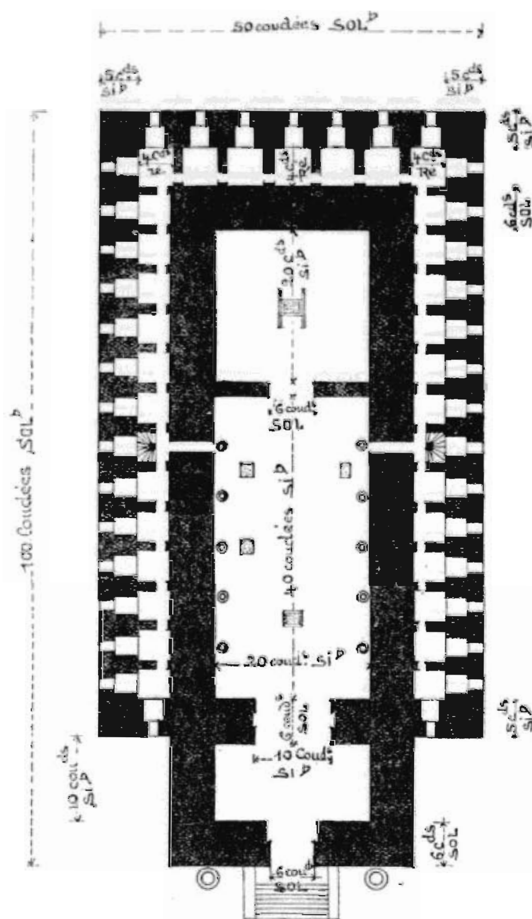
32 coudées Ré EZÉCHIEL. Chapitre XL. Temple.
